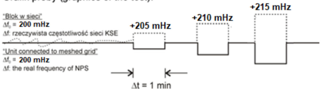
Rys.1 Sprawdzenie niewrażliwości odpowiedzi częstotliwościowej
