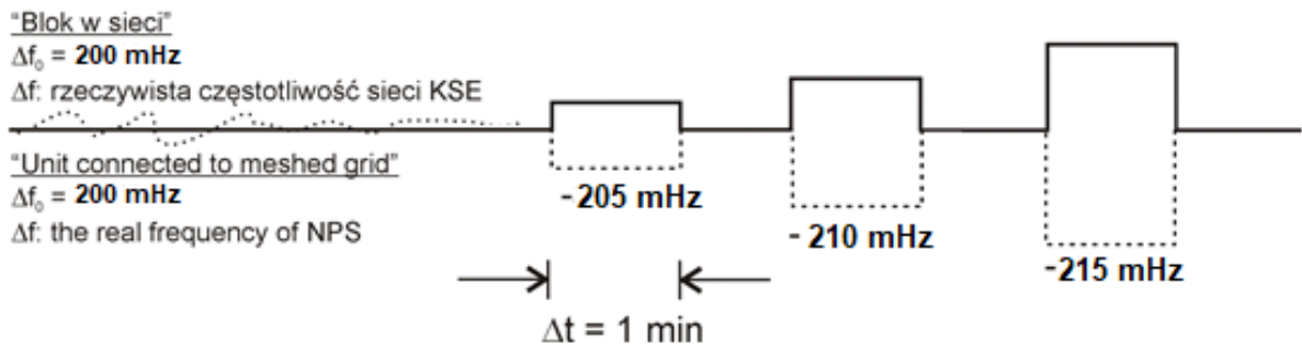
Rys.1 Sprawdzenie niewrażliwości odpowiedzi częstotliwościowej
