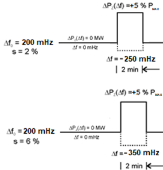
Rys. 2 Sprawdzenie odpowiedzi częstotliwościowej PGM w reakcji na symulowaną pełną zadaną odpowiedź częstotliwościową przy przykładowych ustawieniach statyzmu
