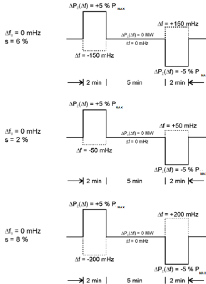
Rys.1 Sprawdzenie odpowiedzi częstotliwościowej PGM w reakcji na symulowaną pełną zadaną odpowiedź częstotliwościową przy różnych ustawieniach statyzmu
