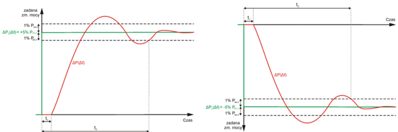
Rys. 2 Kryterialne czasy oceny odpowiedzi częstotliwościowej
