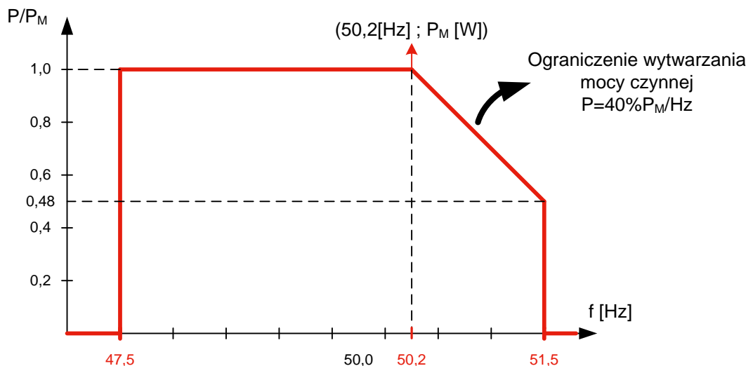
Rys.1 Wymagana charakterystyka P=f(f) wytwarzania mocy czynnej mikroinstalacji i małej instalacji podczas zmian częstotliwości w sieci dystrybucyjnej nN
