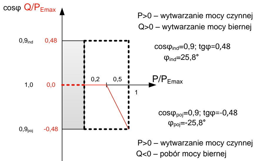
Rys.3 Standardowa charakterystyka \cos\varphi(P) dla źródeł o mocach osiągalnych P_{E_{max}} powyżej 13,8kW
