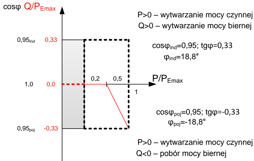
Rys.2 Standardowa charakterystyka \cos\varphi(P) dla źródeł o mocach osiągalnych P_{E_{max}} od 3,68kW do 13,8kW
